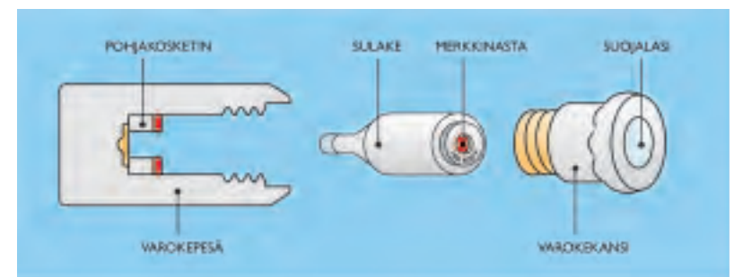
TULPPASULAKKEEN JA VAROKEPESÄN RAKENNE.
