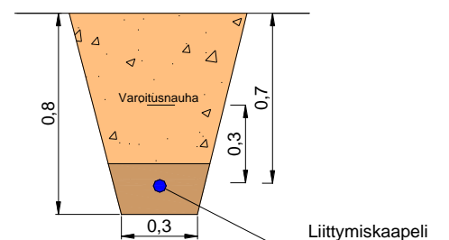
Kuva 2. Kaapeliojan poikkileikkaus.
